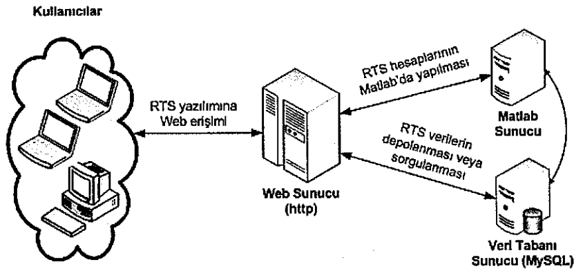
Şekil 1. Web tabanlı soğutma yükü hesaplama uygulaması diyagramı
