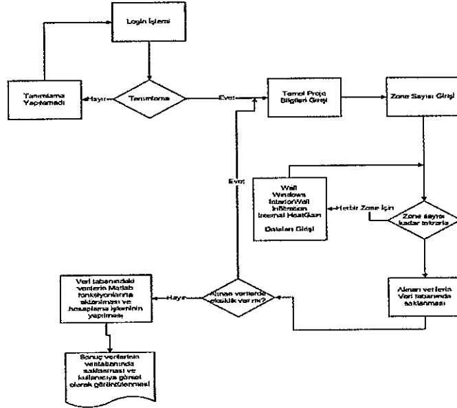
Şekil 2. Geliştirilen programın çalışma algoritması
