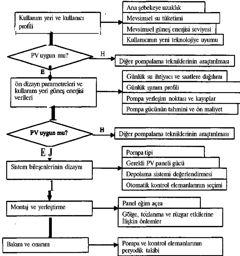
Şekil 2. PV Sistemli Pompa Dizaynının Uygulanma Aşamalarının Blok Diyagram İle Gösterilmesi
