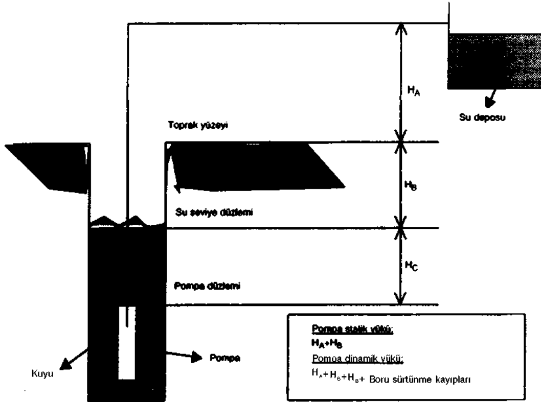
Şekil 3. Pompa Hidrolik Yüküne Etki Eden Faktörlerin Şematik Gösterimi
