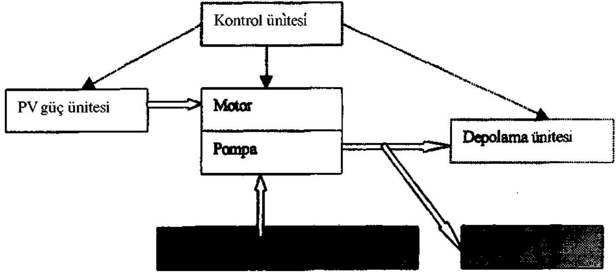
Şekil 1. PV Pompa Sistemi Bileşenlerinin Blok Diyagramı
