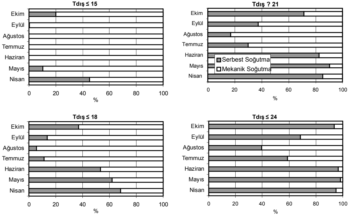
Şekil 7. İzmir ilinin T_{dış} \leq 15^\circ\text{C} , 18^\circ\text{C} 21^\circ\text{C} ve 24^\circ\text{C} şartları için aylık serbest soğutma potansiyelleri
