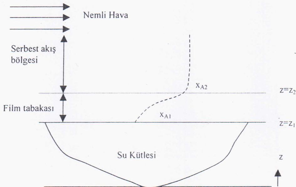
Şekil 1. Kütle transferi mekanizmasının şematik gösterimi.
