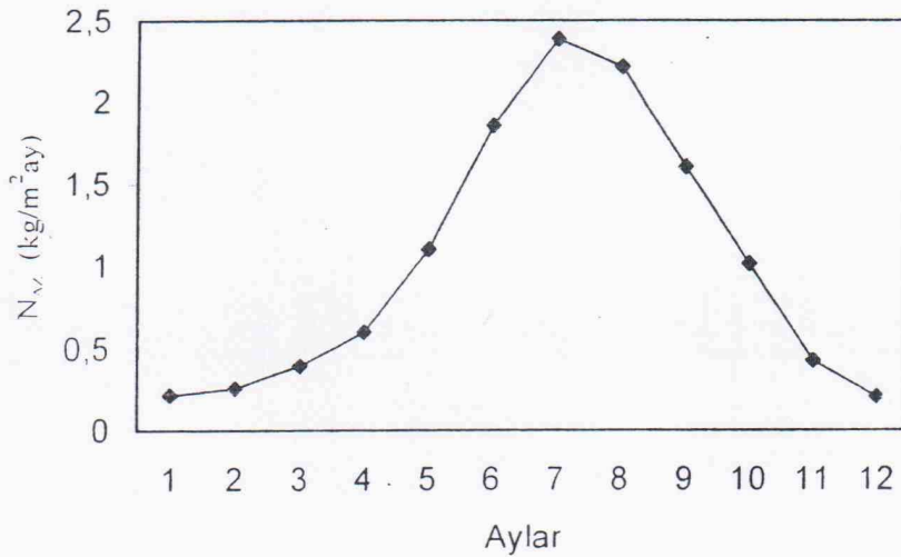
Şekil 3. Denklem (7) ile birim film kalınlığı için ( z_2 - z_1 = 1\text{m} ) hesaplanan aylık buharlaşma miktarı değerleri.
