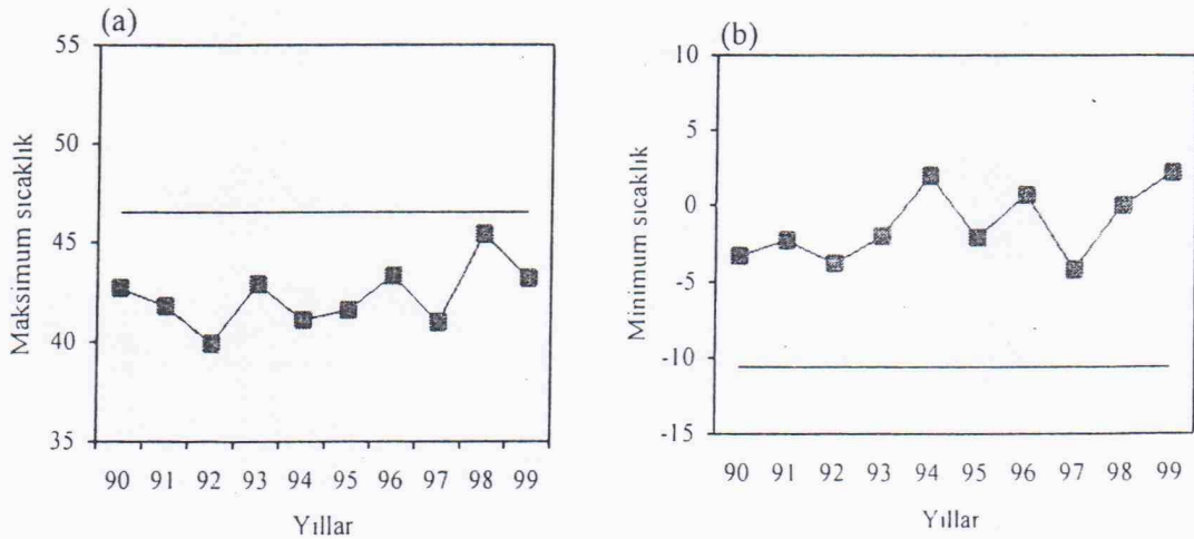
Şekil 4. Baraj sonrası sıcaklık trendinin baraj öncesi uzun yıllar ortalamasıyla belirlenmiş değerle (sürekli çizgi) kıyaslanması; a) maksimum sıcaklık (Temmuz ayı için), b) minimum sıcaklık (Ocak ayı için).
