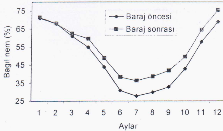
Şekil 2. Şanlıurfa ili baraj öncesi ve baraj sonrası aylık ortalama bağıl nem değerleri.
