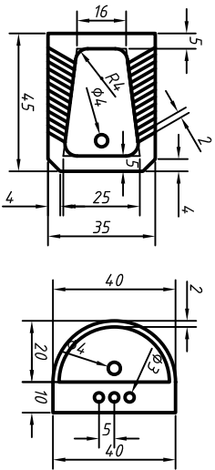
TUVALET TAŞI (fizgi kalınlığı 0.5mm (10p))
