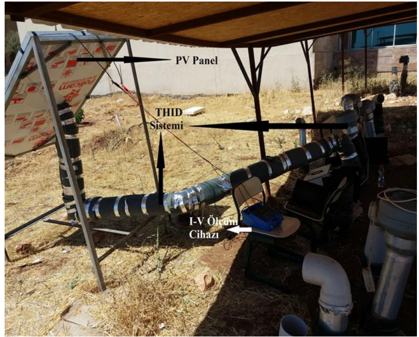
Şekil 4. PV panele montajı yapılan ara parça, PV Panel, THID sistemi ve ölçüm cihazının gösterimi
