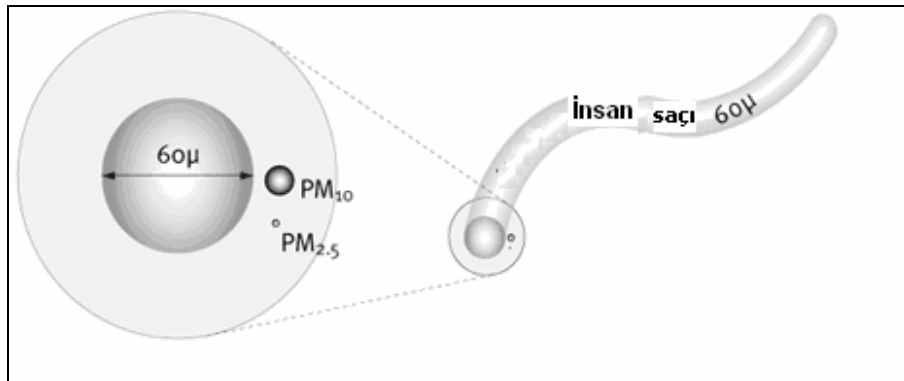
Şekil 3. Partikül maddelerin insan saçına göre boyutları
