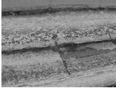
Şekil 10. Urfa ana kanalında yanmış ve çatlamış beton kaplaması
