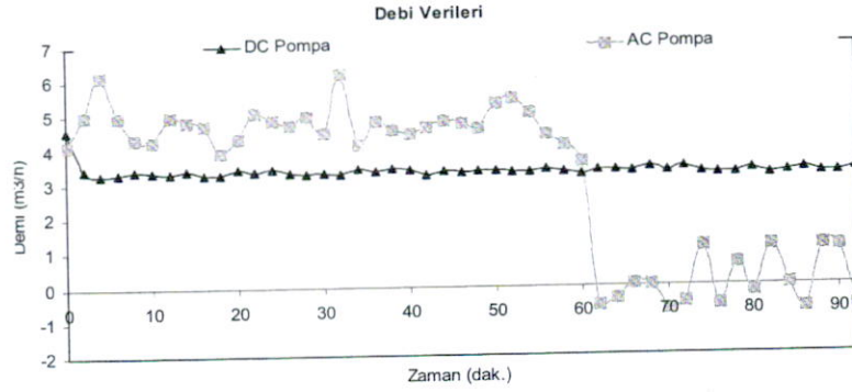
Şekil 3. Gerçek arazi koşullarında yapılan sulamada; a) güç tüketimleri, (b) pompalanan su debileri.
