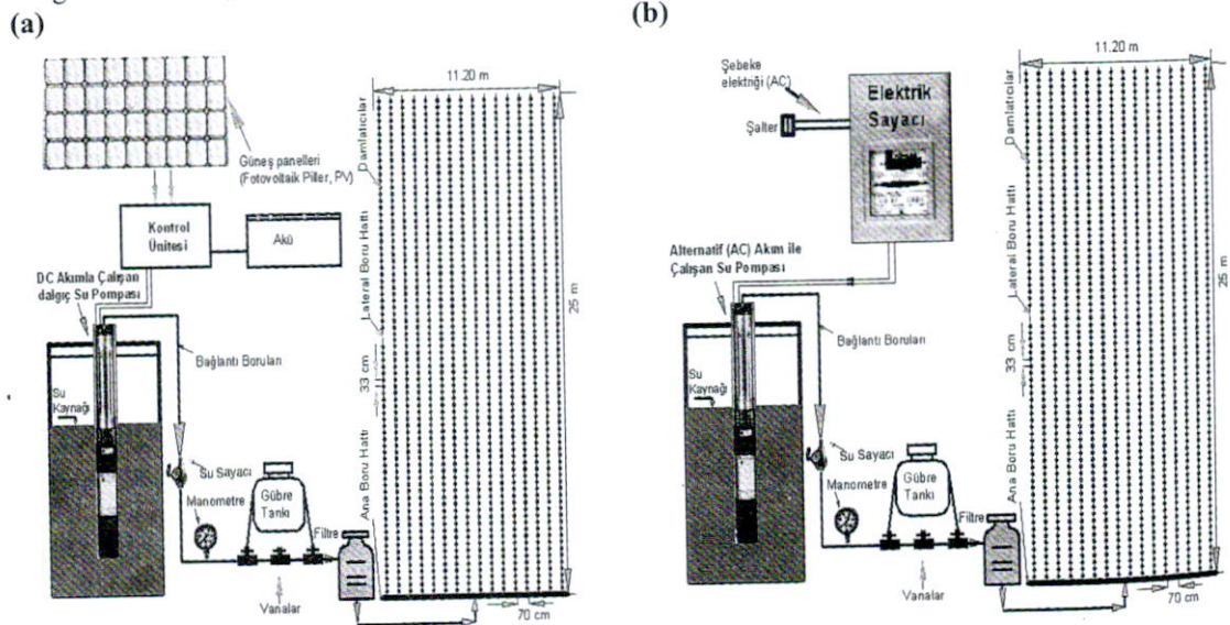
Şekil 1. Sulama sistem ve ekipmanlarına ait şematik şekiller (a) PV-DSS, (b) AC-DSS.
