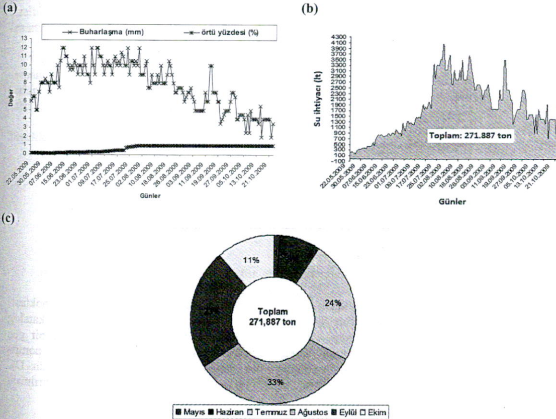
Şekil 2. (a) Buharlaşma ve örtü yüzdesi ölçümleri, (b) Günlük su ihtiyacı, (c) Araziye pompalanan aylık su miktarları.
